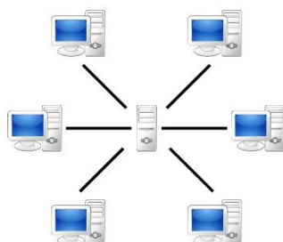
بنية الخادم/العميل
